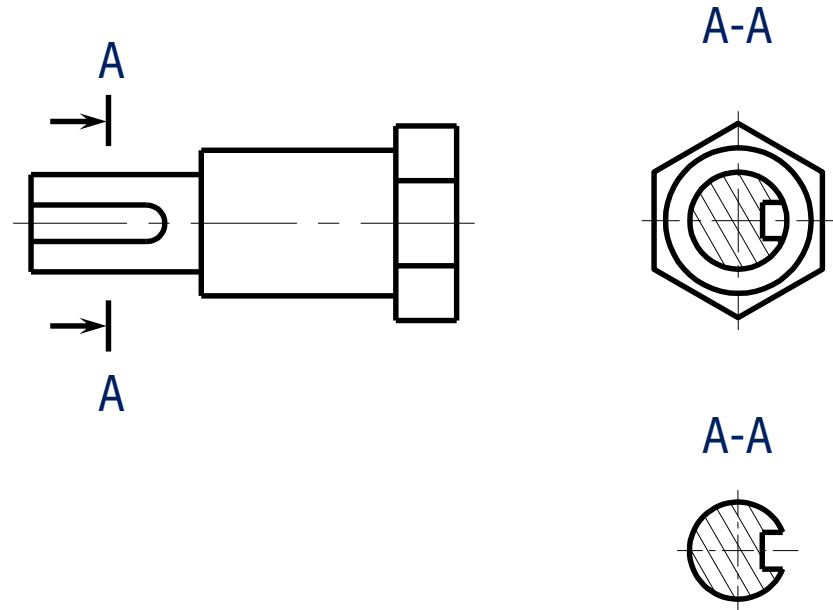
Hình 4.11. Ký hiệu hình cắt và mặt cắt
