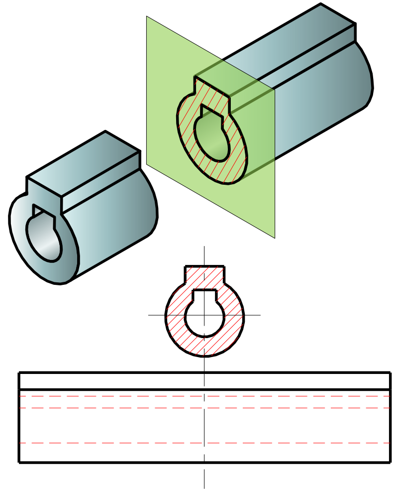
Hình 4.4. Mặt cắt rời
