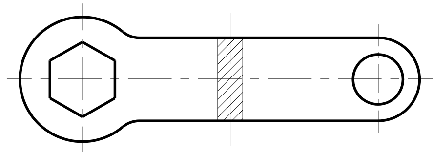
Hình 4.3. Mặt cắt chập
